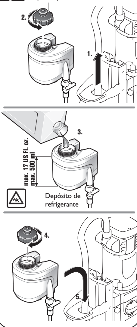
Fig. 4 Tapón superior
