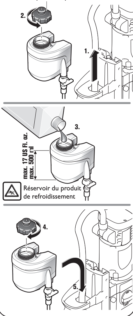
Fig. 4 Capuchon supérieur
