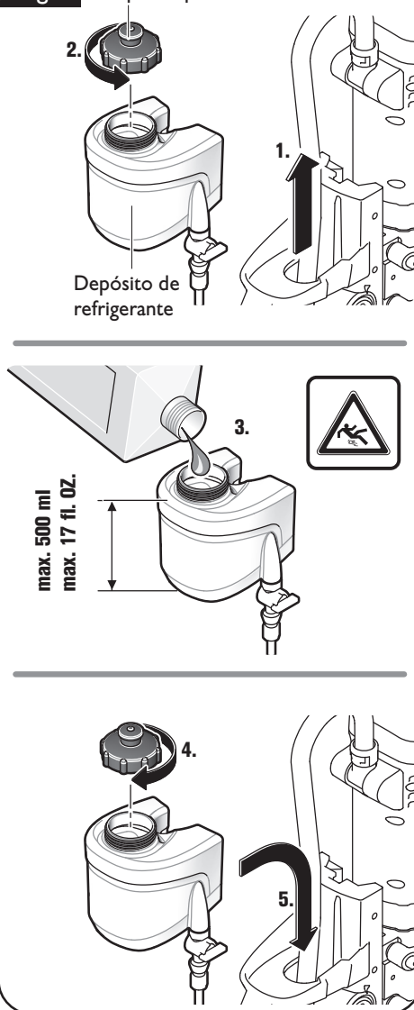
Fig. 5 Tapón superior
