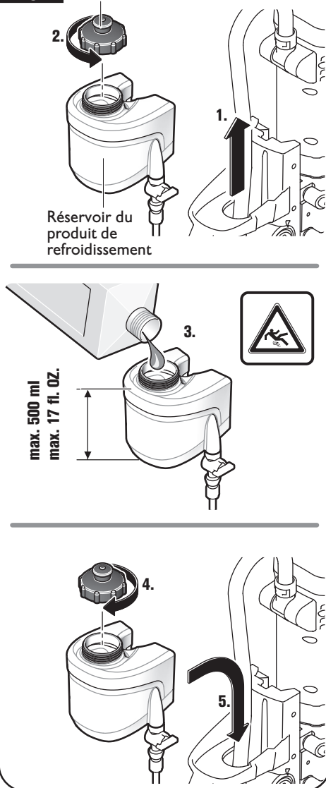
Fig. 5 Capuchon supérieur
